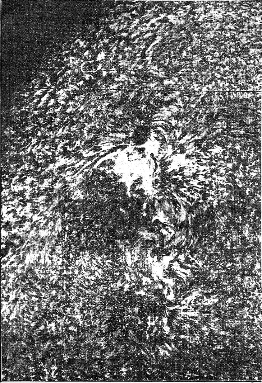
चित्र २३.—सूर्य के भंवर जो विशेष यंत्र से ही देखे जा सकते हैं
